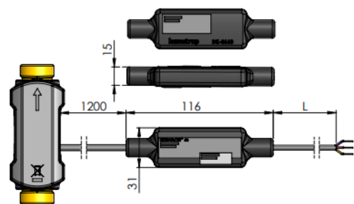
Elektronikbox
