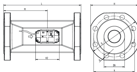
Abmessungen qp 25.0- 100.0
