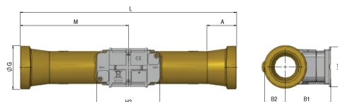
Abmessungen qp 3.5- 10.0
