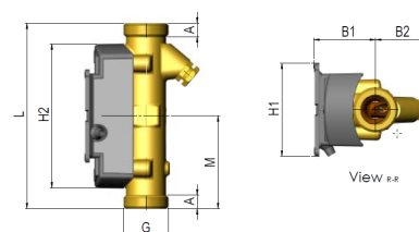
Dimensions qp 1.5- 2.5
