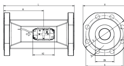
Dimensions qp 25.0- 100.0
