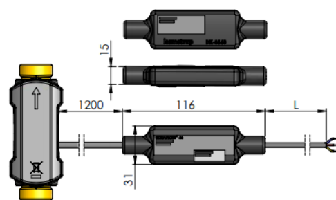
Boîtier électronique
