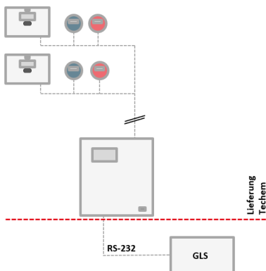
Einbindung über den M-Bus-Master (RS-232)
