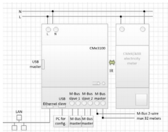
Anschlusschema
