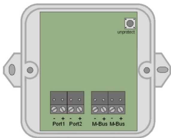
IC-M2 Anschlüsse
