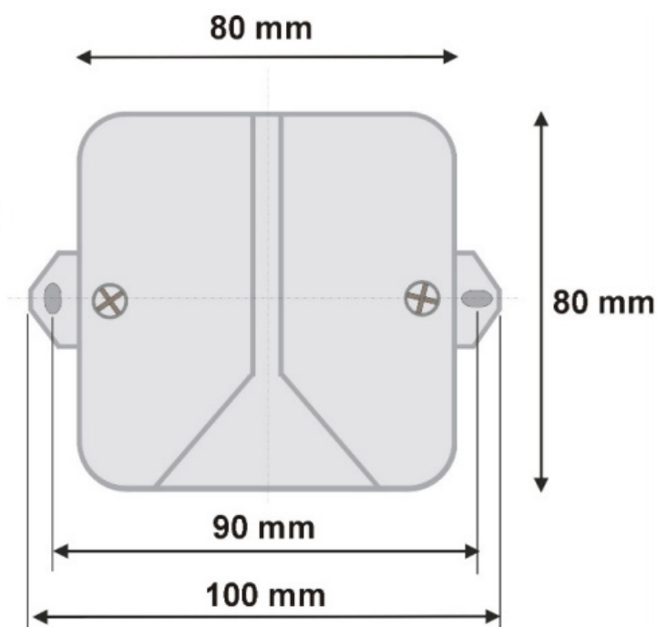
IC-M2 Grundriss vermasset
