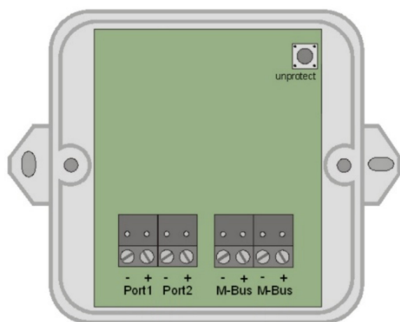
Connexions IC-M2
