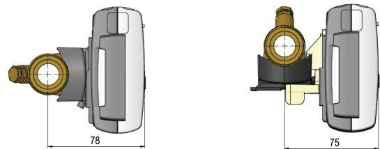
MULTICAL® 603 montiert auf ULTRAFLOW® mit G \frac{3}{4} Gewindeanschluss
