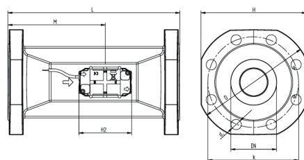
Dimensions qp 25.0- 100.0
