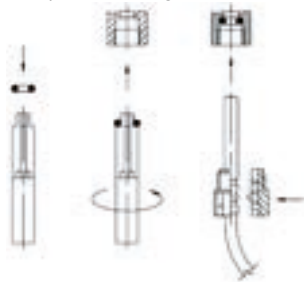
III. 5: Montering af adaptersæt
