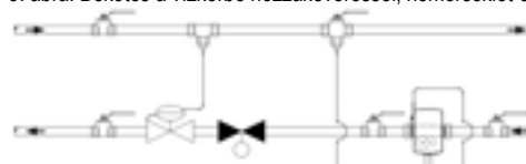
4. ábra: Bekötés a vízkörbe pl. fűtő kapcsolással (az átfolyás-érzékelő a szabályozószelep / nyomáskülönbség-szabályzó előtt)
