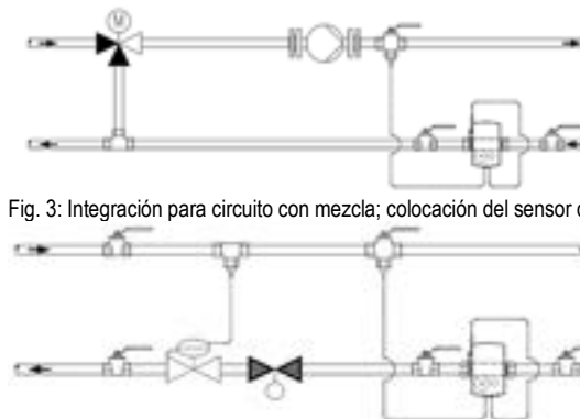
Fig. 3: Integración para circuito con mezcla; colocación del sensor de temperatura
