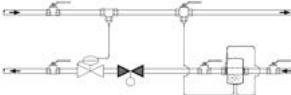
Fig. 4: Montaj pentru circuit, de exemplu, cu drosel (senzor debit în direcția de curgere înainte de supapa de reglare / regulatorul de presiune diferențială)
