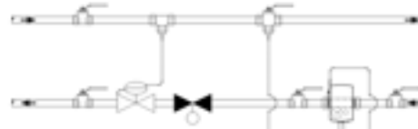
Fig. 4: Allacciamento per circuito con ad es. strozzamento (sensore di portata in direzione del flusso a monte della valvola regolatrice/del regolatore della pressione differenziale)
