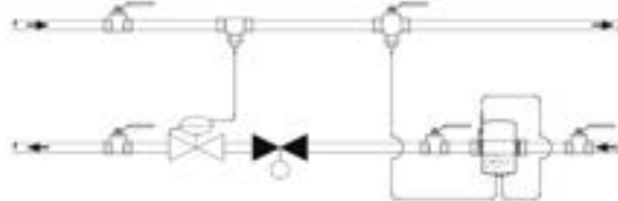
III. 4: Montering til kredsløb med f.eks. drosselkobling (gennemstrømsmåler i flowretning før reguleringsventil/differenstrykregulator)
