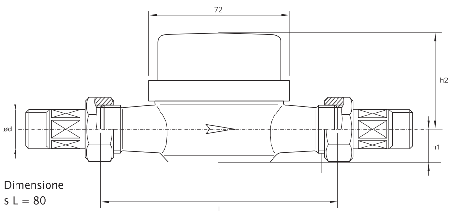
Dimensiones del contador de agua
