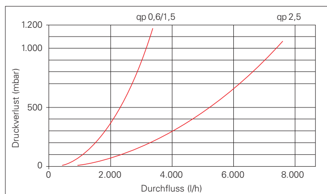
Druckverlustdarstellung 4.5.2
